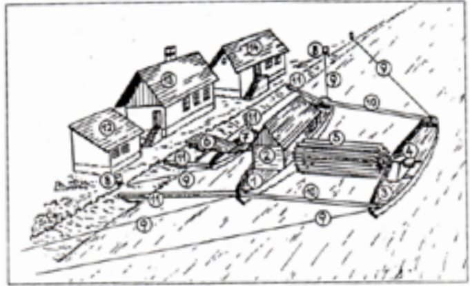
Skizze einer Schiffsmühle 1)
