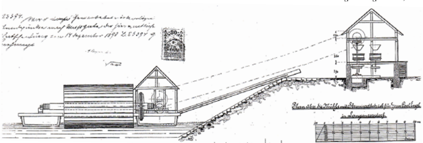
Abb. 1: Technische Zeichnung der Engl-Mühle, 1898
